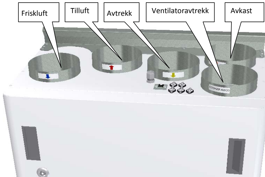
(Skisse viser AHU-200 V)
