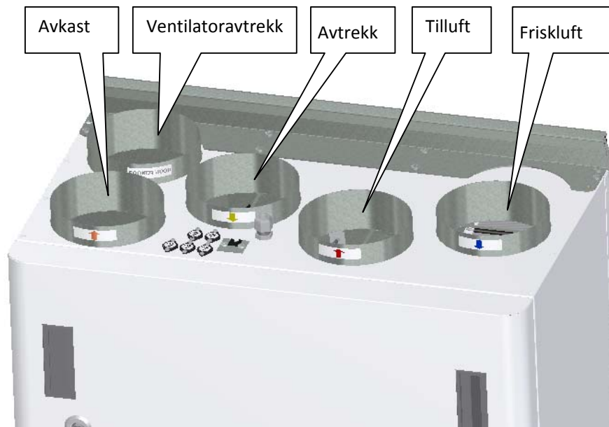
(Skisse viser AHU-200 H)
