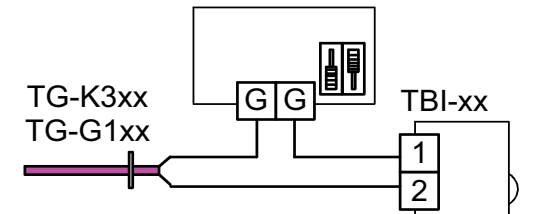
Fig. 6: Emplacement des switches et branchements pour contrôle d'ambiance et utilisant séparément une sonde externe et une TBI-xx comme point de consigne.*
