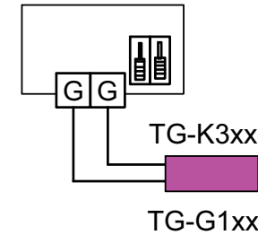
Fig. 3: Emplacement des switches et branchements pour consigne interne et sonde externe.*
