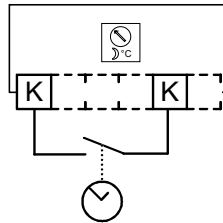
Abb. 7: Einschalten der Nachtabsenkungsfunktion.
