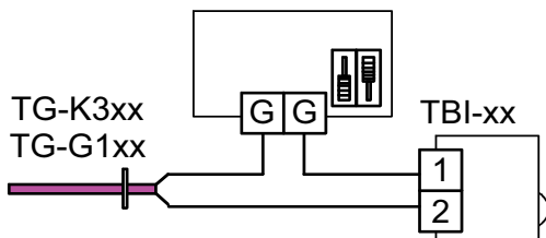
Abb. 6: Umschalter und Anschluß an externem, separatem Fühler und Potentiometer TBI-xx als SollwertEinstellung*
